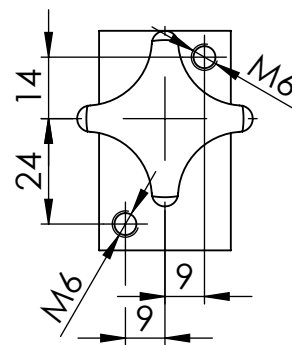
Ansicht/View X4
